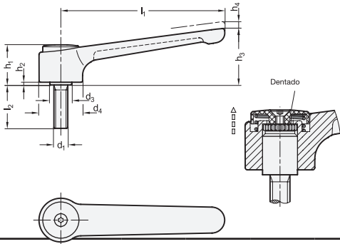
GN 126.1-Espárrago roscado
